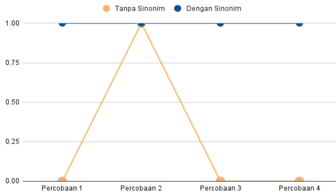
Gambar 4. 1 Grafik Bleu Skor Dengan dan Tanpa Sinonim
